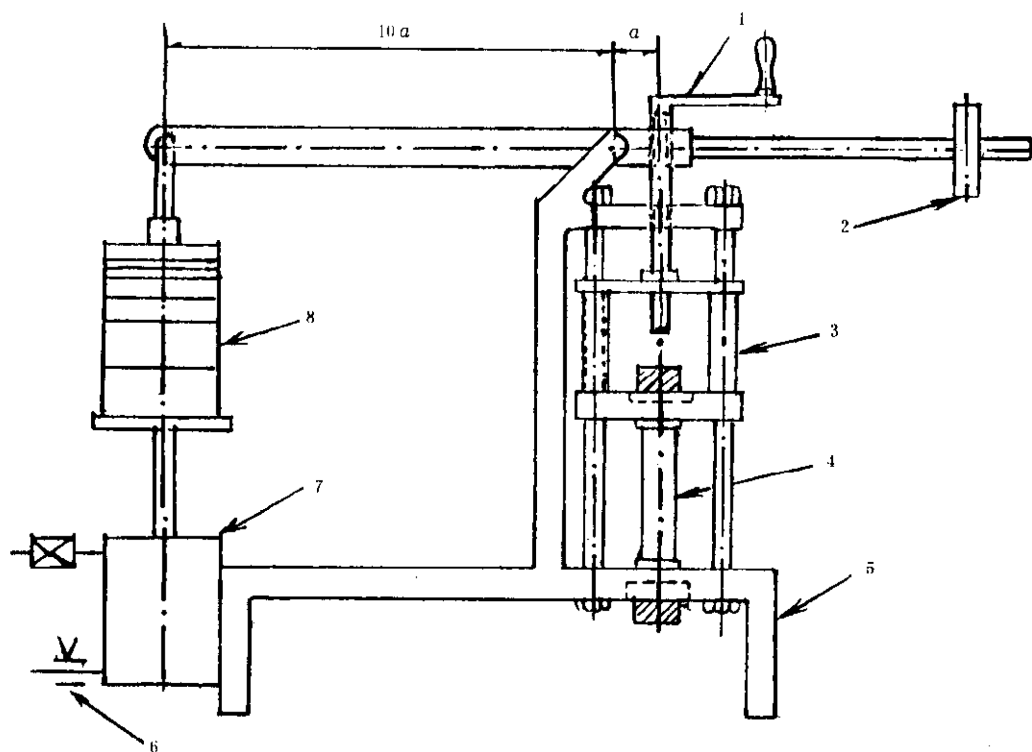
图1 拉力计简图
